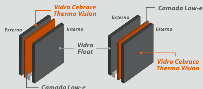
Figura 2: Cebrace Thermo Vision aplicado na Refrigeração.
